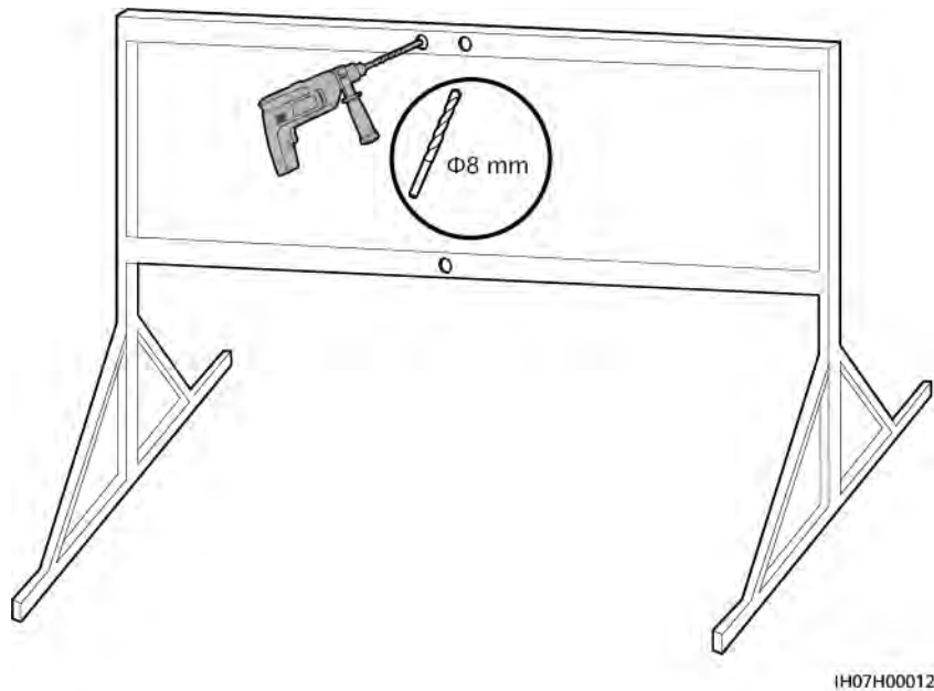
Figura 4-14 Taladrado de los orificios
