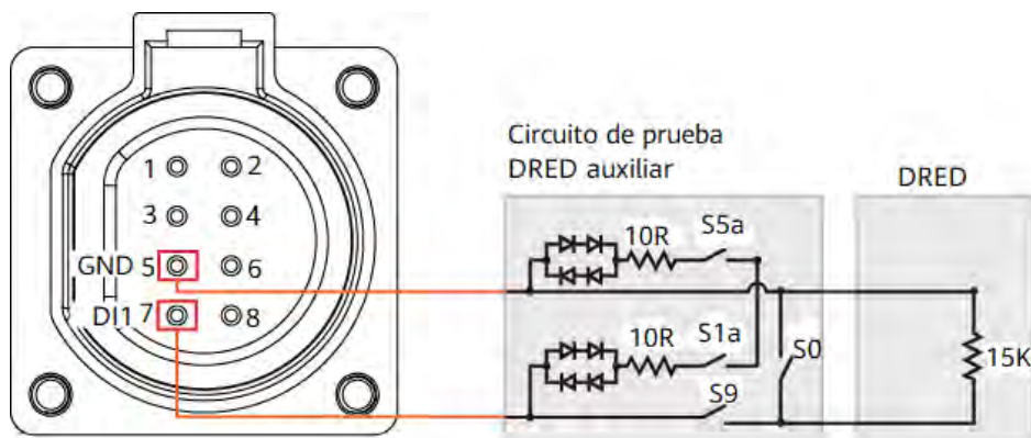
Figura 7-16 Diagrama de cableado de la función DRM
