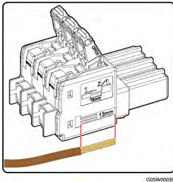
Figura 5-9 Longitud para el pelado de cables
